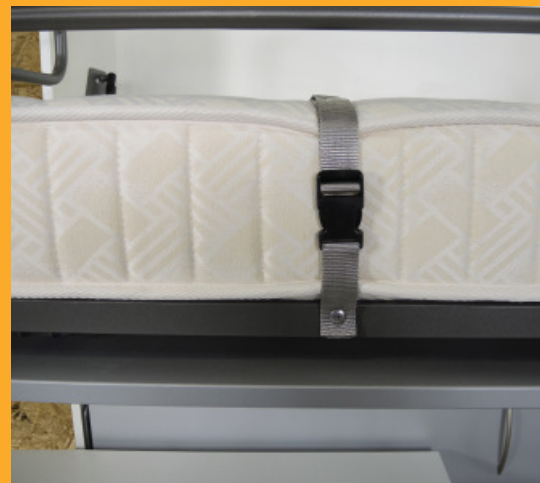
2 2 sangles clipées et réglables retiennent chaque matelas lors de la manoeuvre du lit
