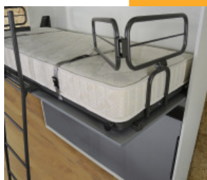
3 Rembardes de sécurité sur le pourtour complet du couchage supérieur, repliables sur le matelas, avec blocage sur l'échelle
